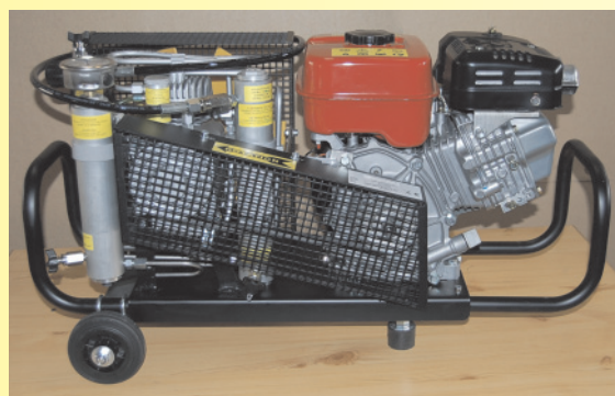
Obr. č. 29 kompresor Benda MK 120 benzin
